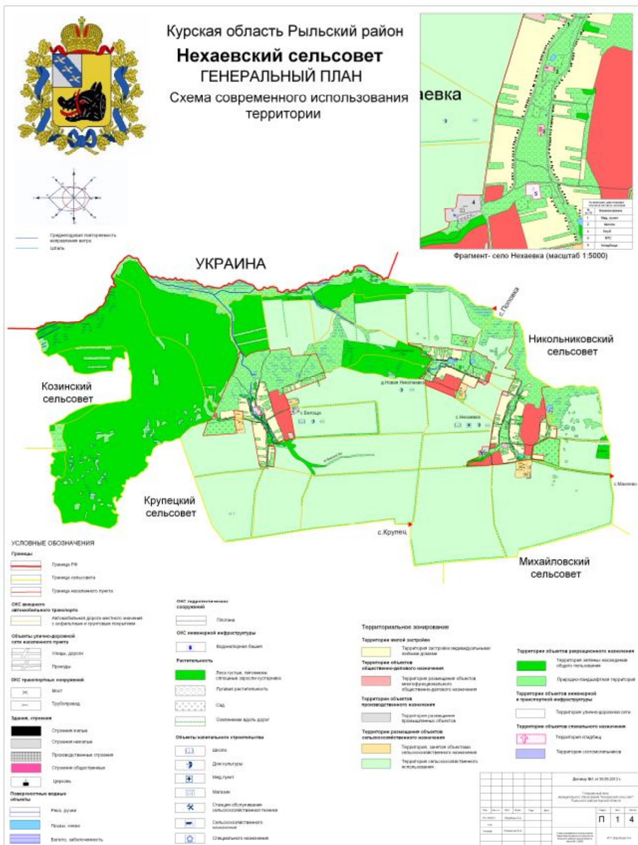
Рис.1. Генеральный план (Схема современного использования территории) муниципального образования «Нехаевский сельсовет» Рыльского района Курской области.
